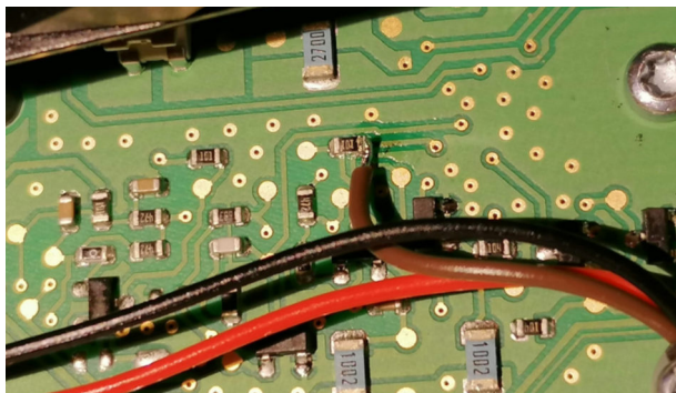
Abbildung 7: Anschlussbereich (oben) und Anschlusspunkt (unten).
