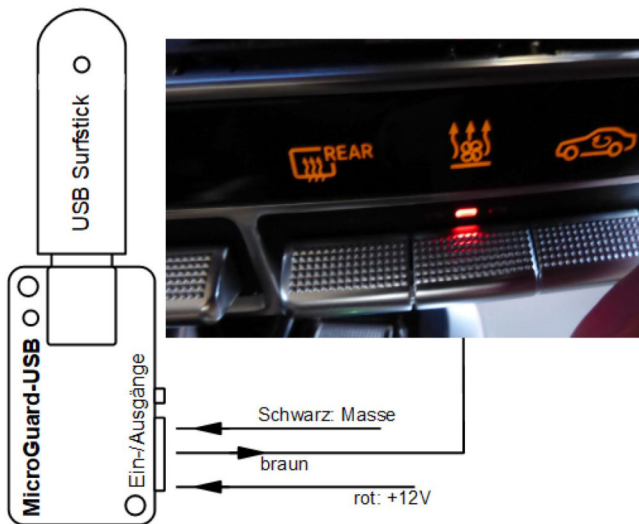
Abbildung 2: Standheizungsschalter im Mercedes V-Klasse Baureihe 447-2
