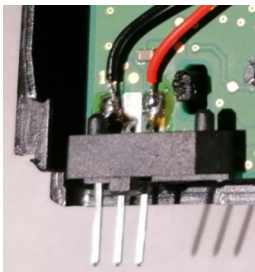
Abbildung 8: Anschluss der Spannungsversorgung für das Modul
