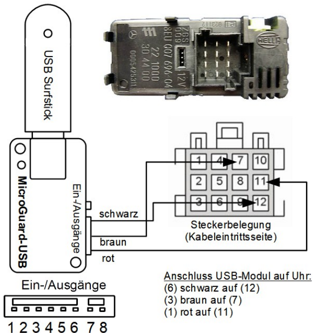
Abbildung 2: Anschluss des MicroGuard-USB Moduls an die Leitungen zur Moduluhr. Anschluss an PIN7 entspricht der Funktion des externen Tasters (Uhr steuert die Heizung)
