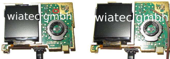
Abbildung 4: Platine Vorwahluhr MultiControl und der Anschlusspunkt
